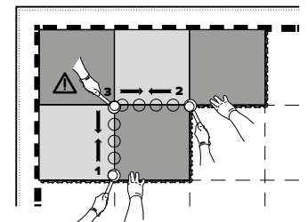
Abb. 4: Verlegungsmethode der Fliesen ROBUST invisible , ROBUST design
