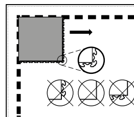
Abb. 3: Verlegungsrichtung der Fliesen ROBUST invisible , ROBUST design
