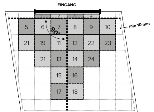
Abb. 1: Verlegung ROBUST strong , ROBUST strong PLUS , ROBUST XL
